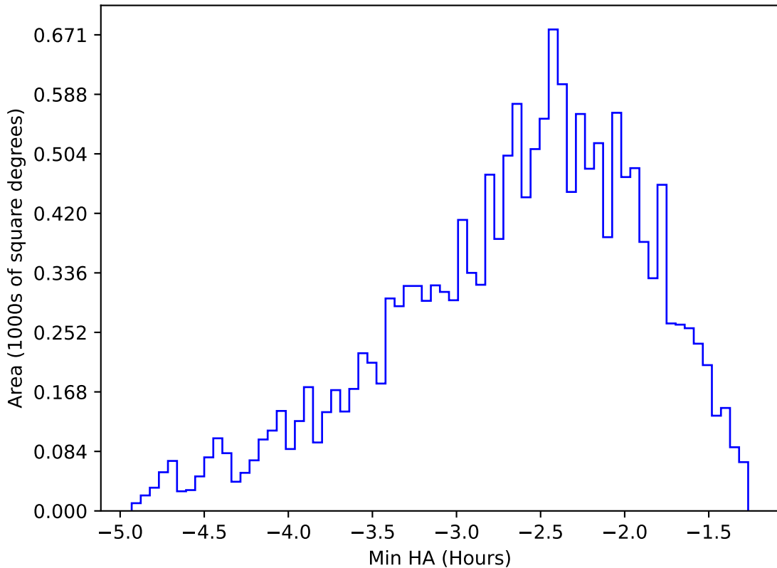
retro_baseline_v2.0_10yrs WFD z band: Min HA
