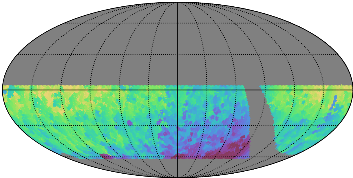
retro_baseline_v2.0_10yrs WFD y band: Min HA
