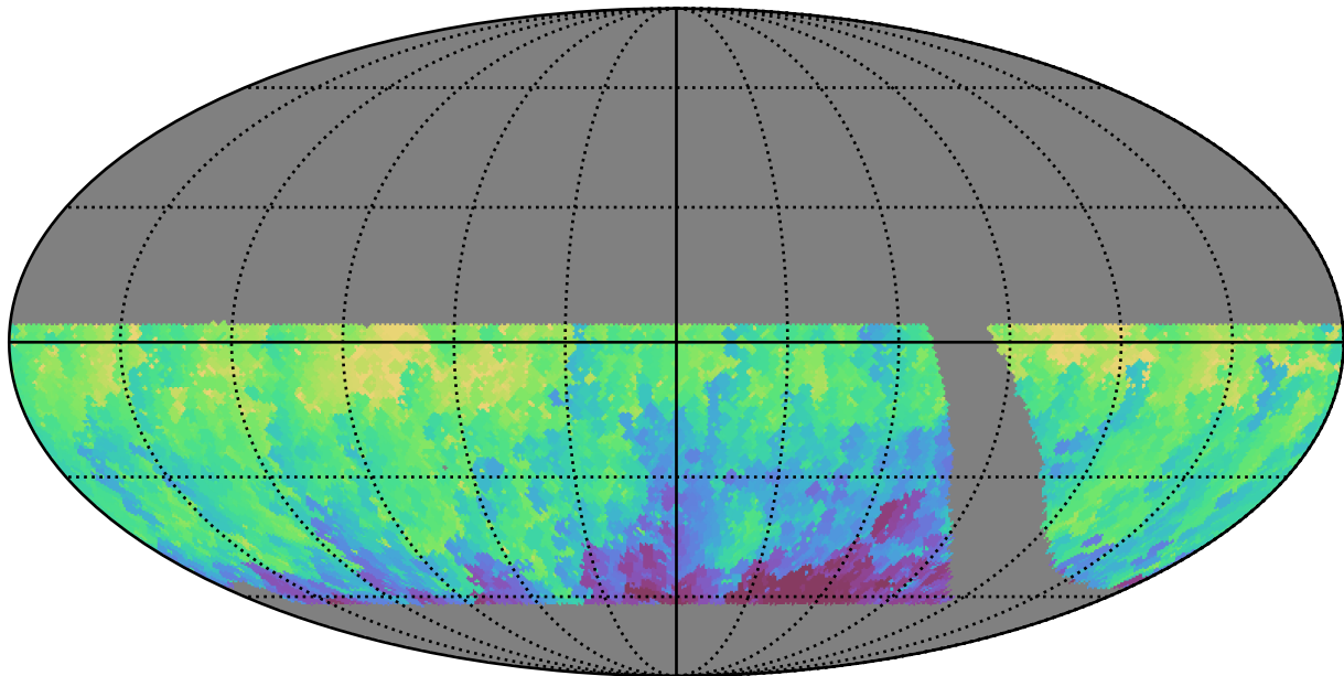
retro_baseline_v2.0_10yrs WFD u band: Min HA
