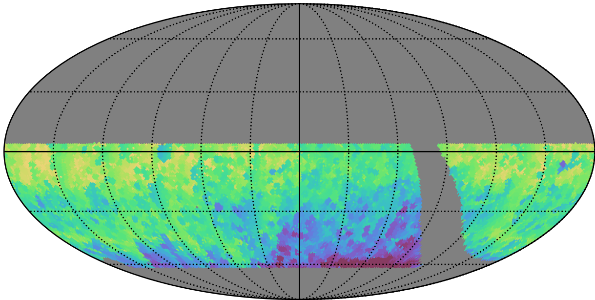
retro_baseline_v2.0_10yrs WFD r band: Min HA
