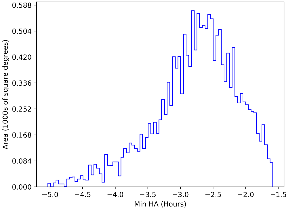
retro_baseline_v2.0_10yrs WFD r band: Min HA
