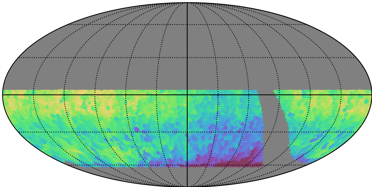
retro_baseline_v2.0_10yrs WFD i band: Min HA
