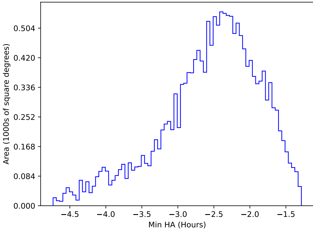
retro_baseline_v2.0_10yrs WFD g band: Min HA
