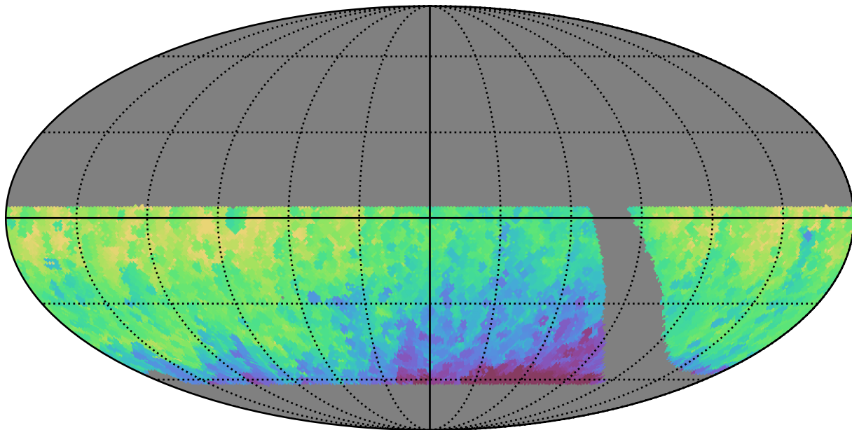
retro_baseline_v2.0_10yrs WFD all bands: Min HA
