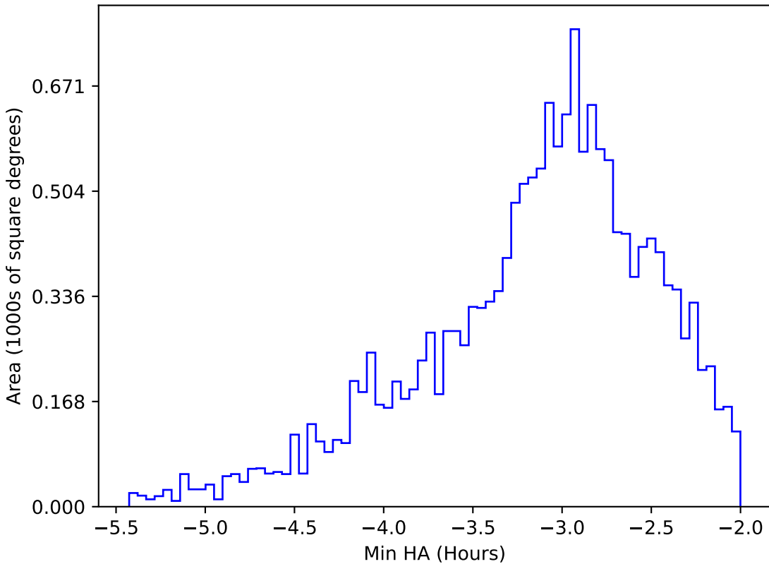
retro_baseline_v2.0_10yrs WFD all bands: Min HA
