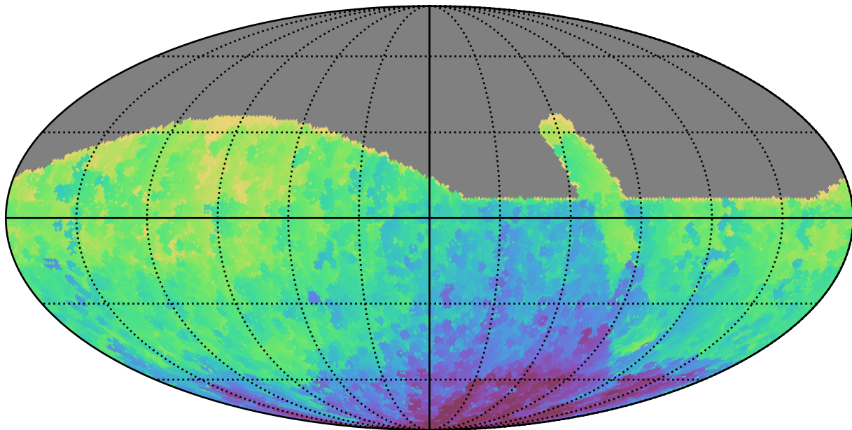
retro_baseline_v2.0_10yrs All sky z band: Min HA
