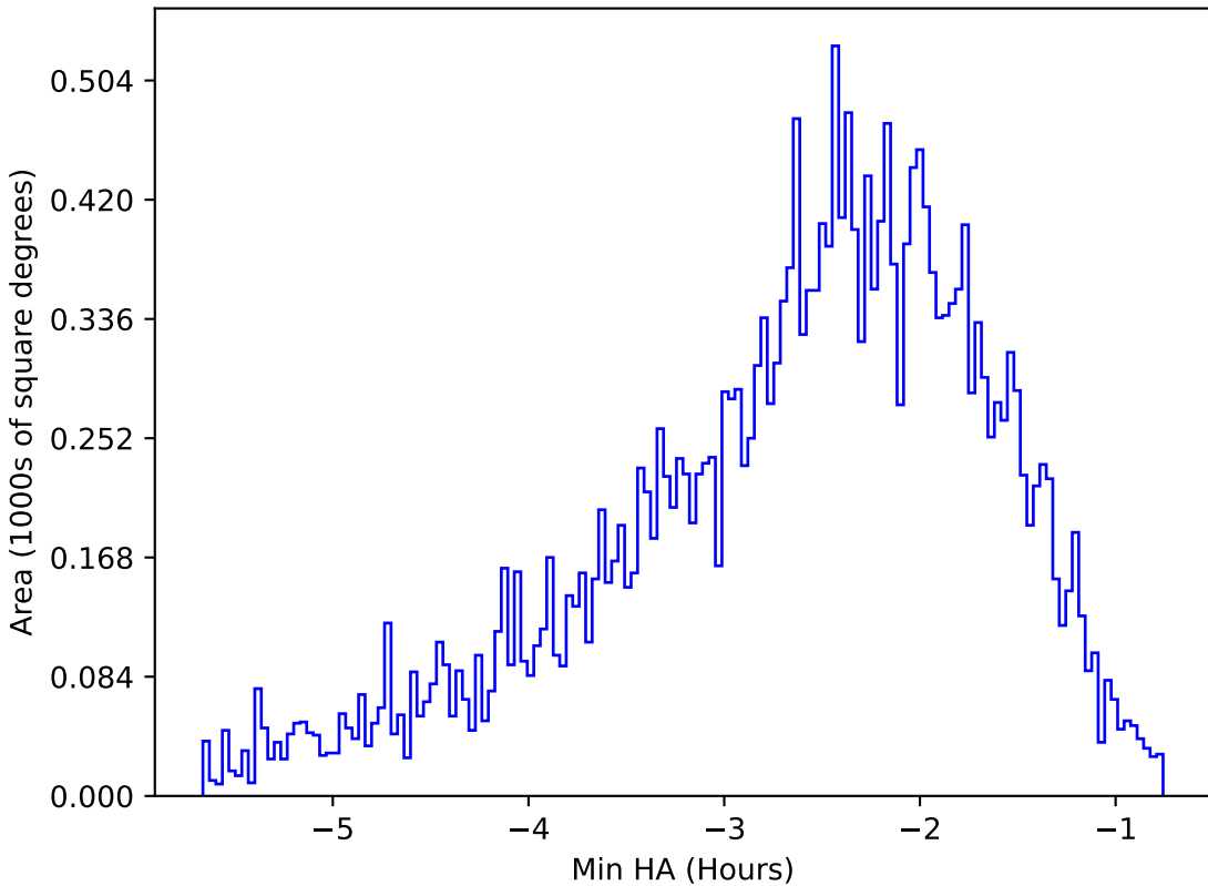
retro_baseline_v2.0_10yrs All sky z band: Min HA
