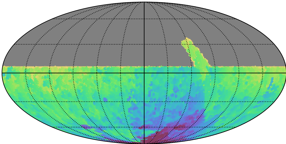
retro_baseline_v2.0_10yrs All sky y band: Min HA
