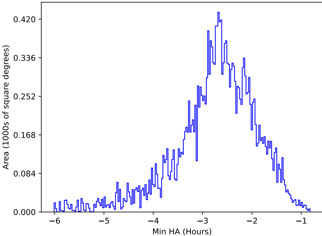
retro_baseline_v2.0_10yrs All sky y band: Min HA
