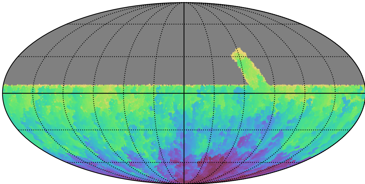
retro_baseline_v2.0_10yrs All sky u band: Min HA
