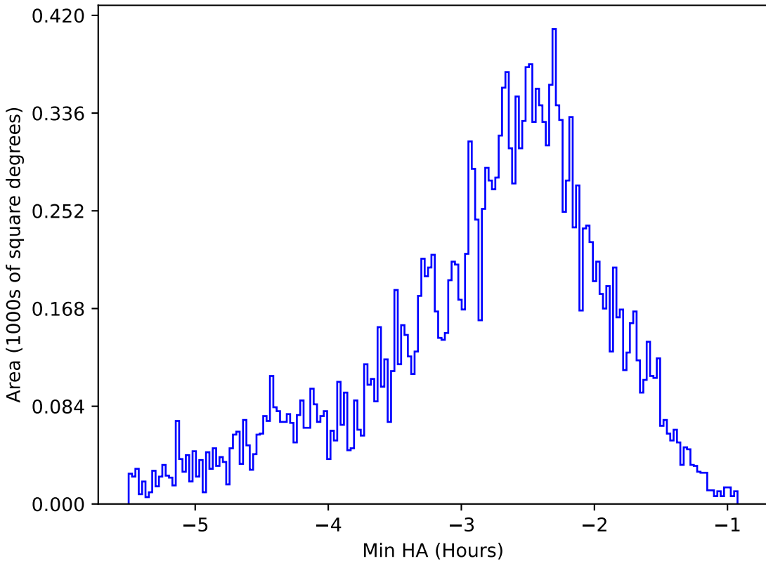
retro_baseline_v2.0_10yrs All sky u band: Min HA
