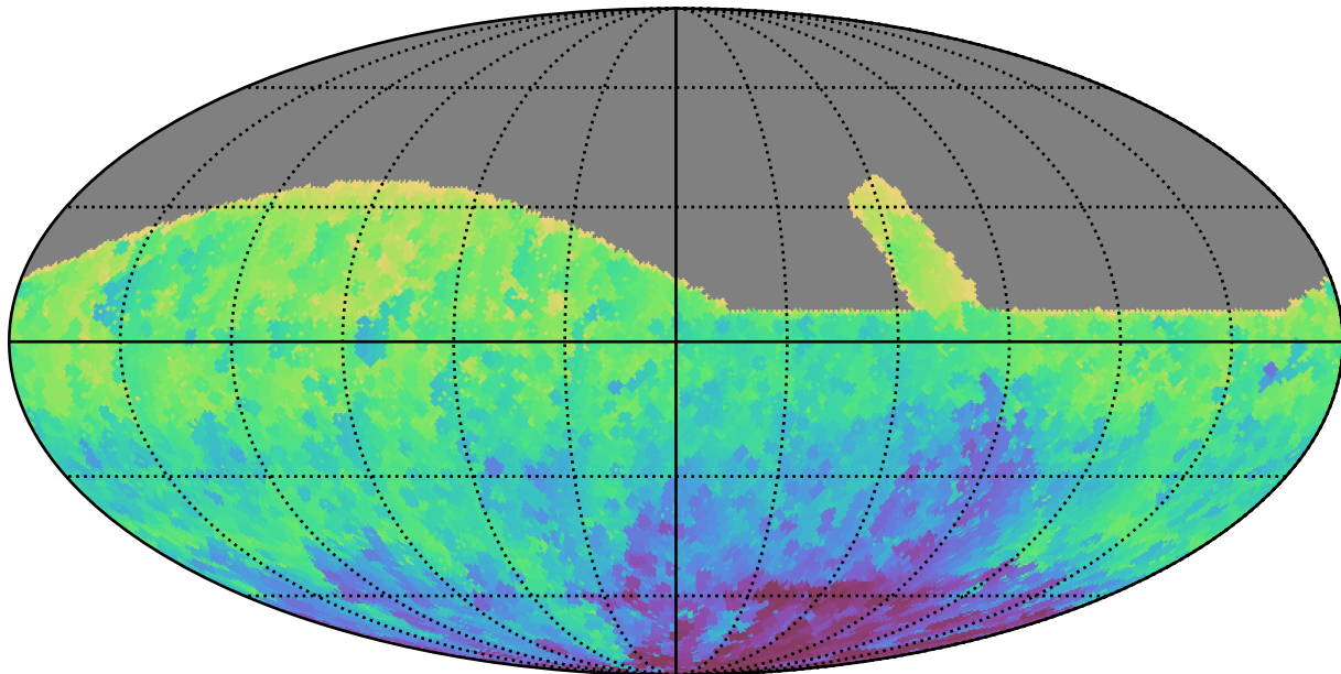
retro_baseline_v2.0_10yrs All sky r band: Min HA
