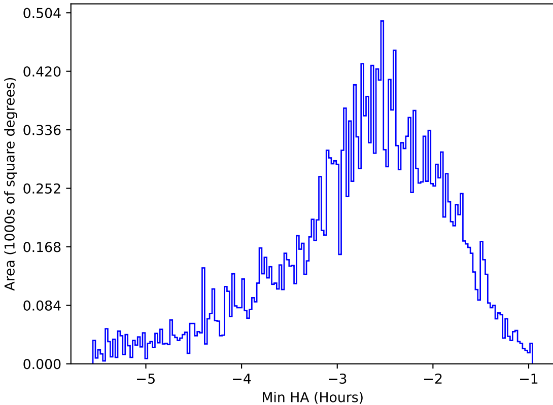
retro_baseline_v2.0_10yrs All sky r band: Min HA
