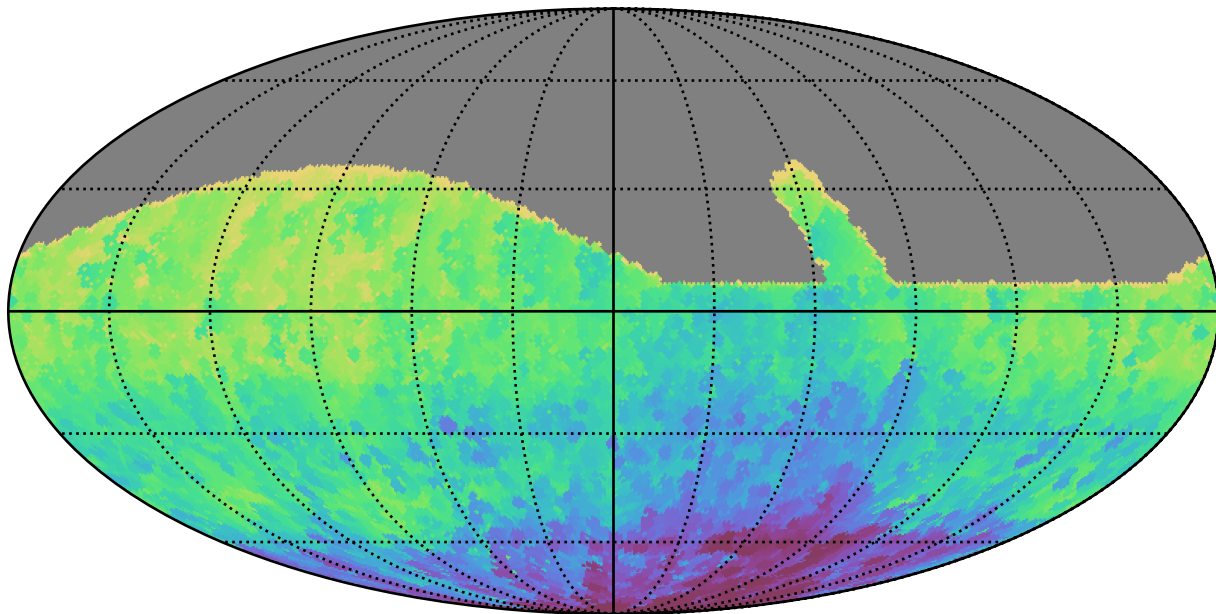
retro_baseline_v2.0_10yrs All sky i band: Min HA
