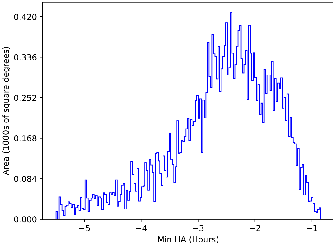
retro_baseline_v2.0_10yrs All sky i band: Min HA
