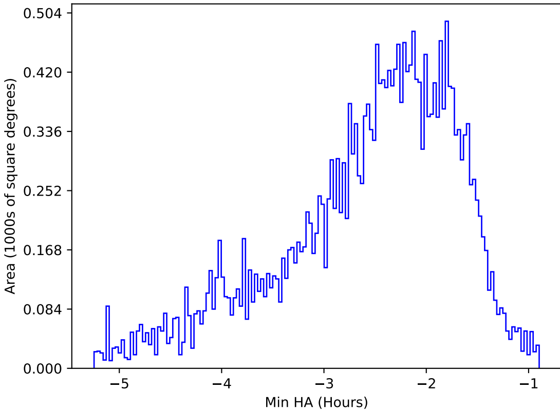
retro_baseline_v2.0_10yrs All sky g band: Min HA
