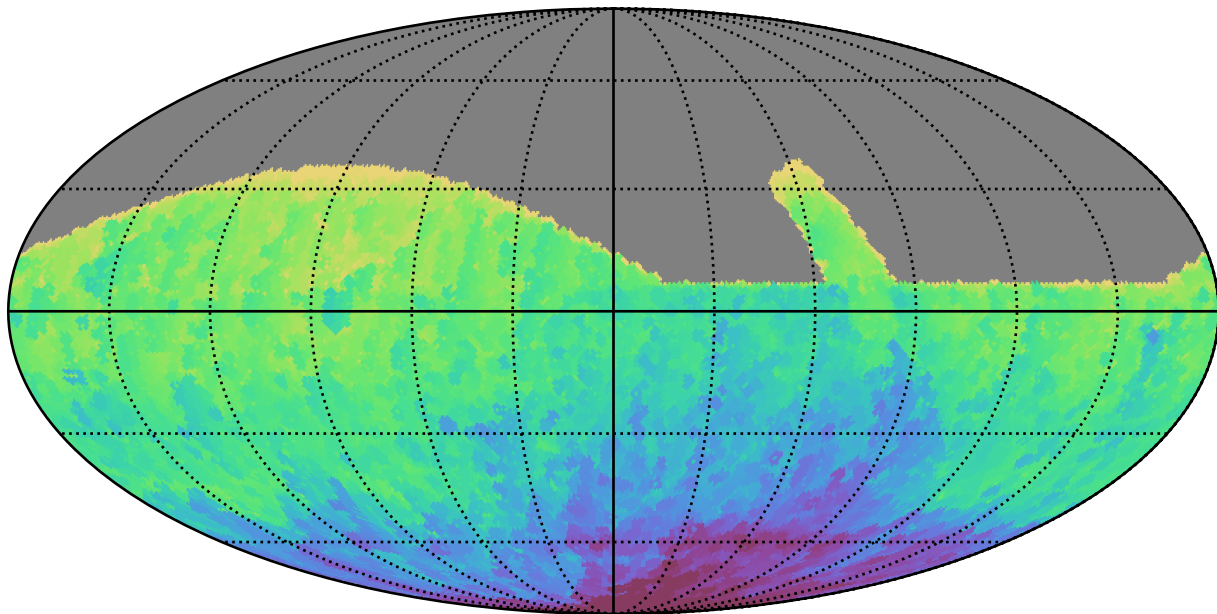
retro_baseline_v2.0_10yrs All sky all bands: Min HA
