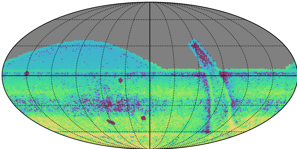
retro_baseline_v2.0_10yrs All sky: Median Intra-Night Gap
