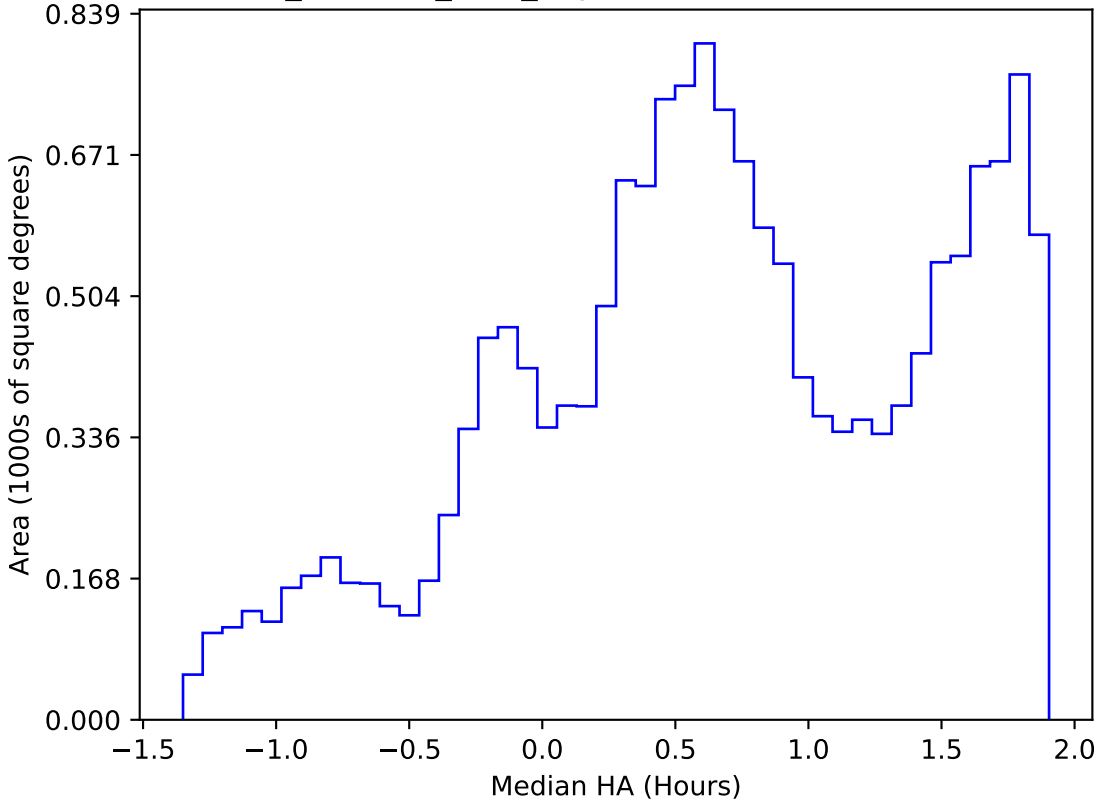
retro_baseline_v2.0_10yrs WFD z band: Median HA
