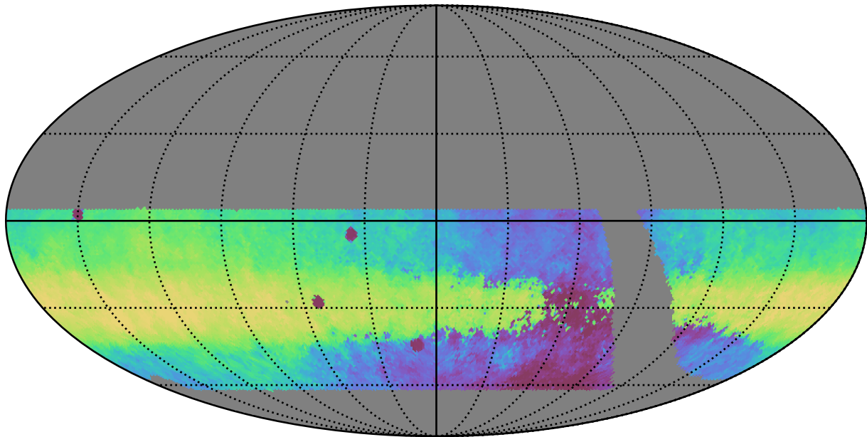
retro_baseline_v2.0_10yrs WFD y band: Median HA
