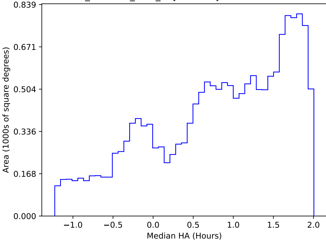
retro_baseline_v2.0_10yrs WFD y band: Median HA
