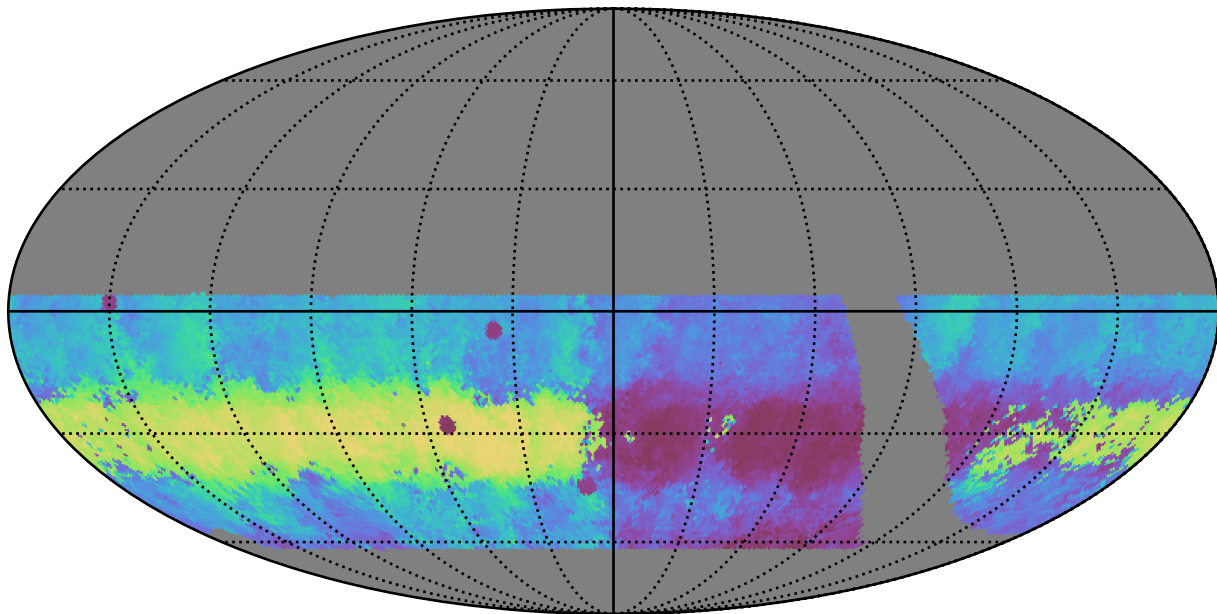
retro_baseline_v2.0_10yrs WFD u band: Median HA
