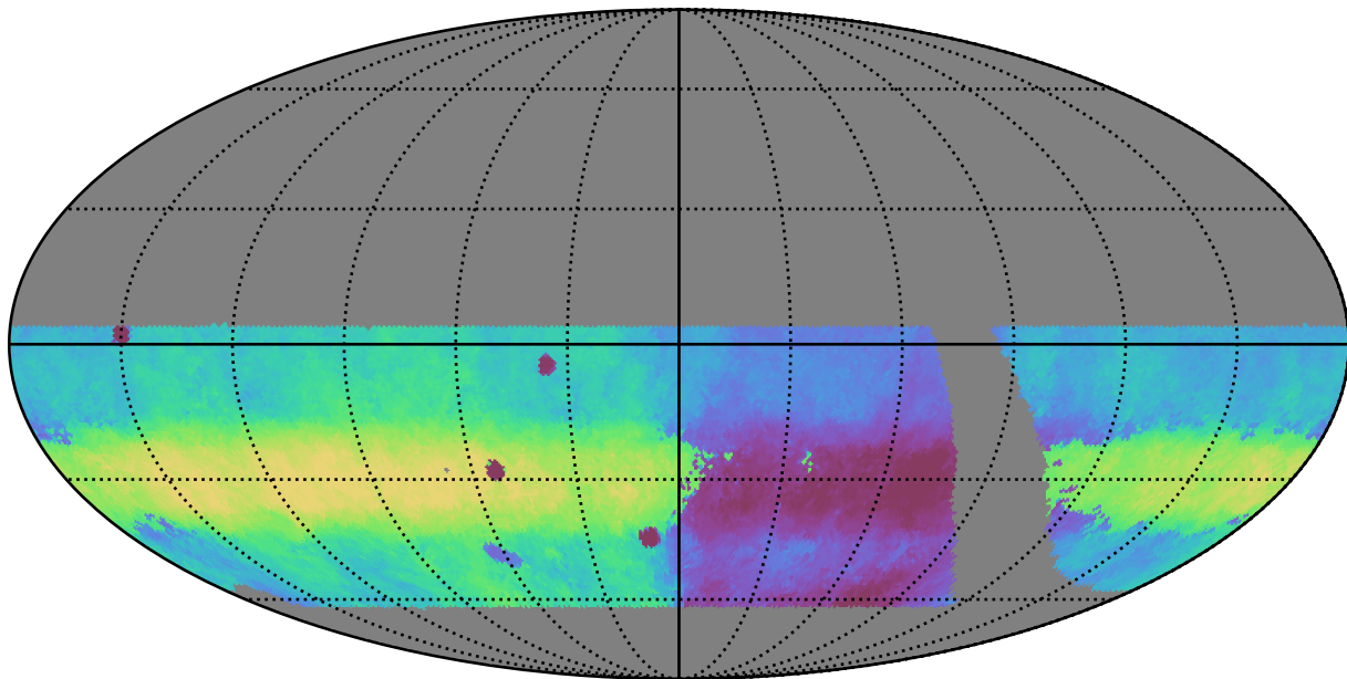
retro_baseline_v2.0_10yrs WFD r band: Median HA
