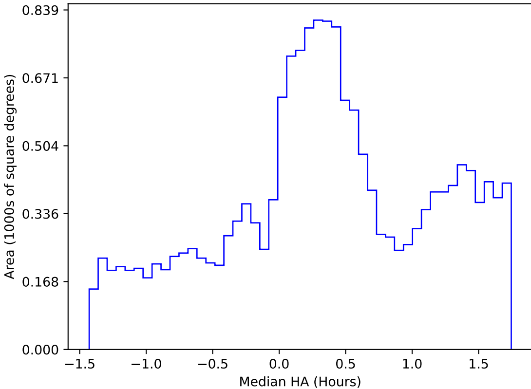
retro_baseline_v2.0_10yrs WFD r band: Median HA
