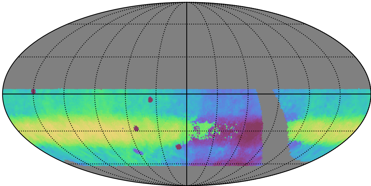
retro_baseline_v2.0_10yrs WFD i band: Median HA
