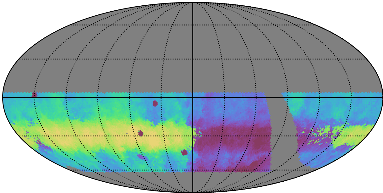
retro_baseline_v2.0_10yrs WFD g band: Median HA
