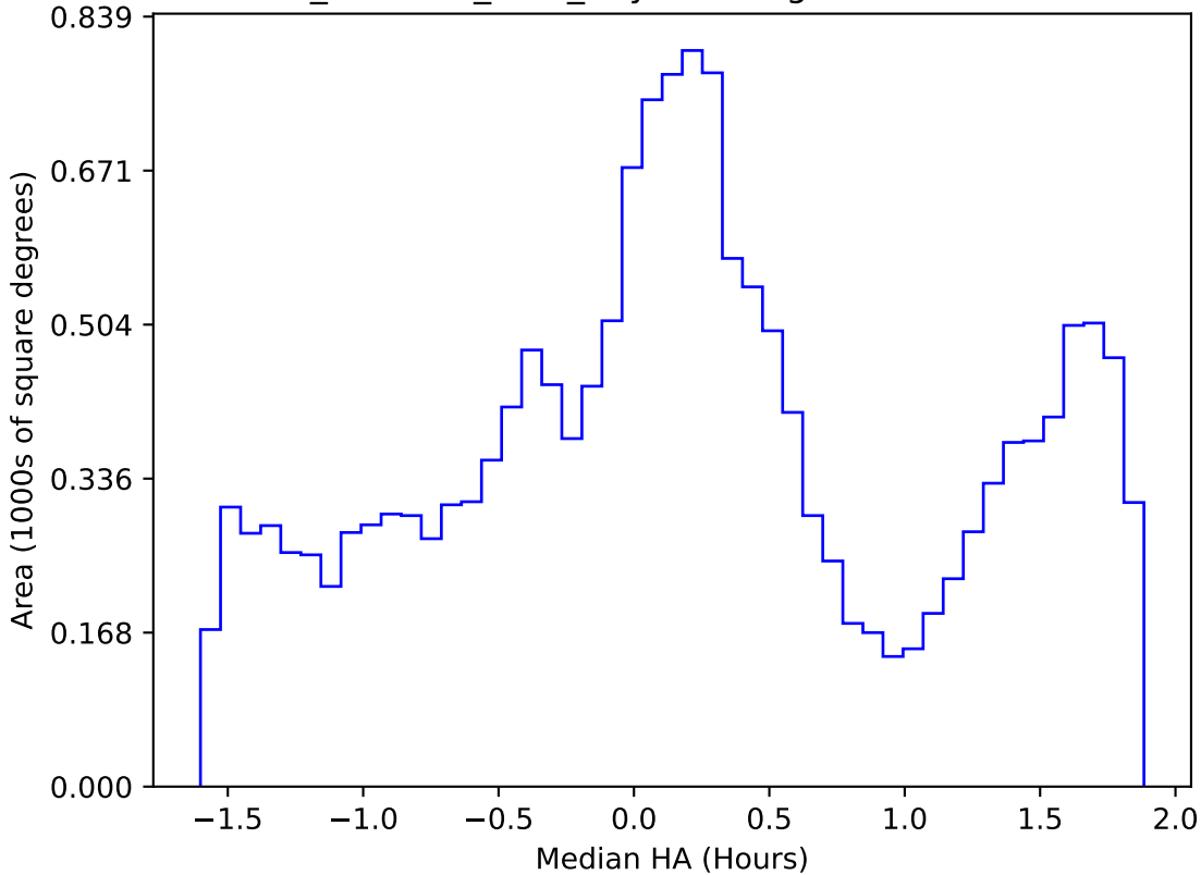
retro_baseline_v2.0_10yrs WFD g band: Median HA
