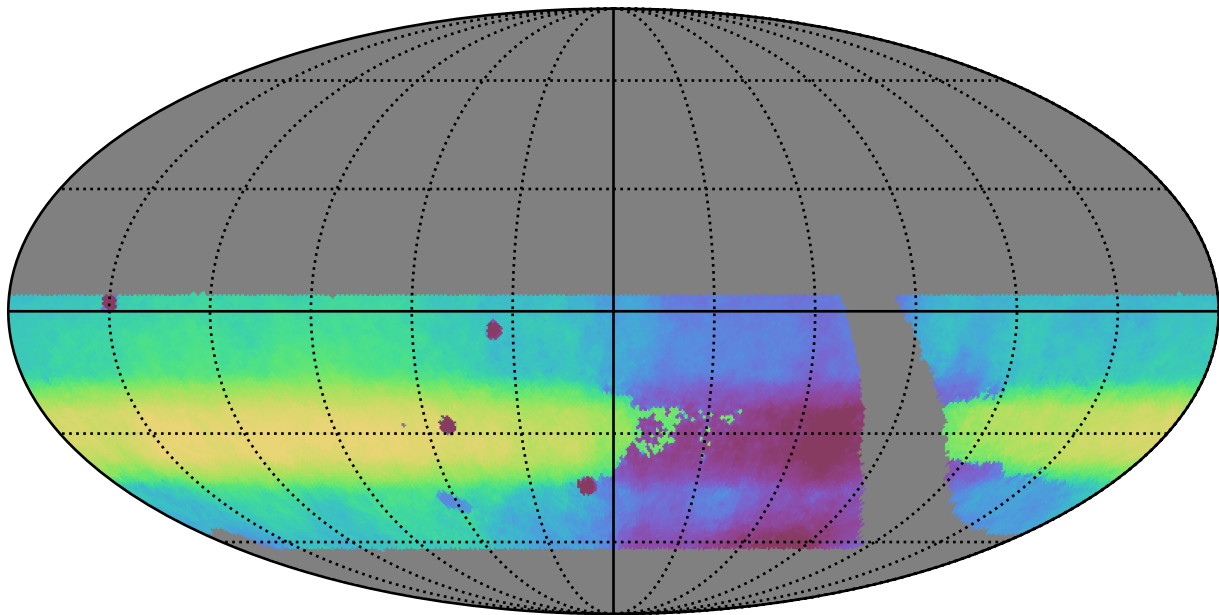
retro_baseline_v2.0_10yrs WFD all bands: Median HA
