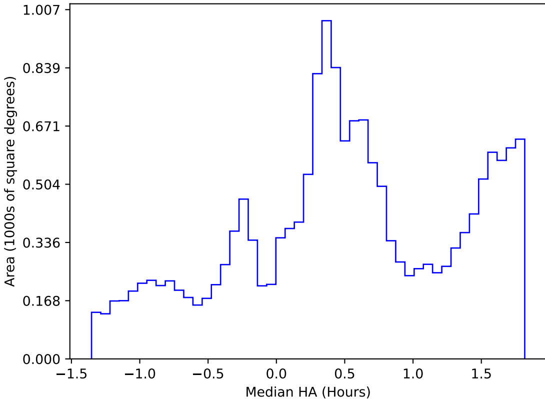
retro_baseline_v2.0_10yrs WFD all bands: Median HA
