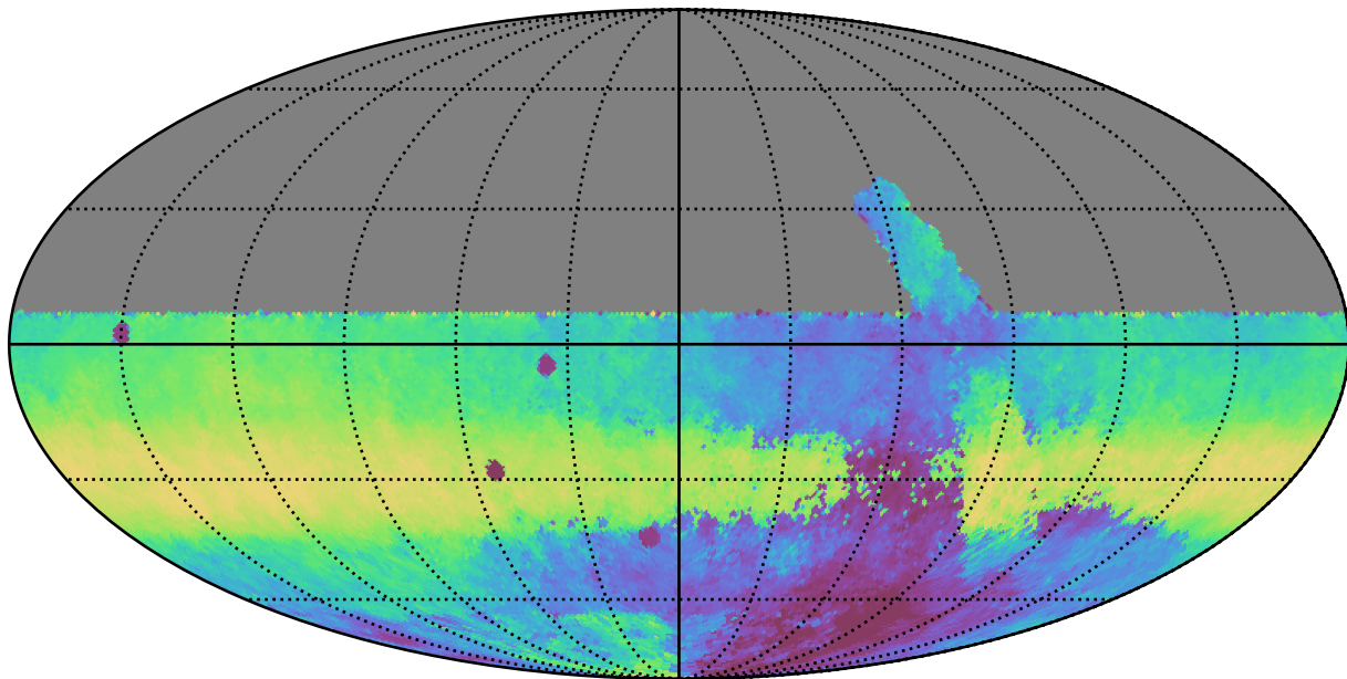
retro_baseline_v2.0_10yrs All sky y band: Median HA
