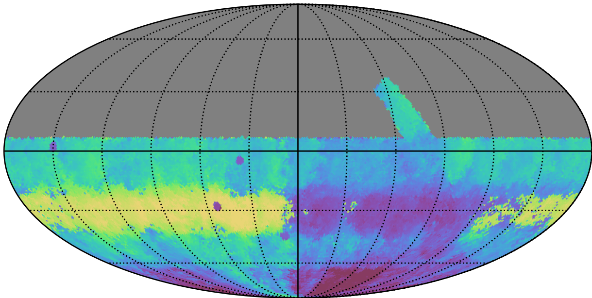
retro_baseline_v2.0_10yrs All sky u band: Median HA
