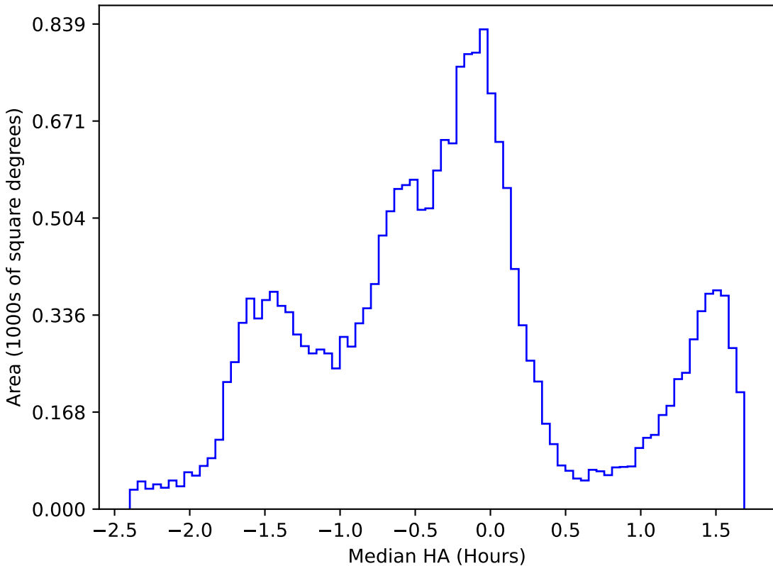
retro_baseline_v2.0_10yrs All sky u band: Median HA
