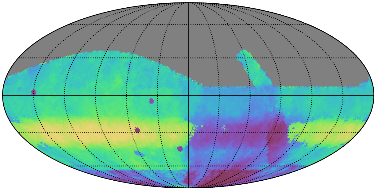
retro_baseline_v2.0_10yrs All sky r band: Median HA
