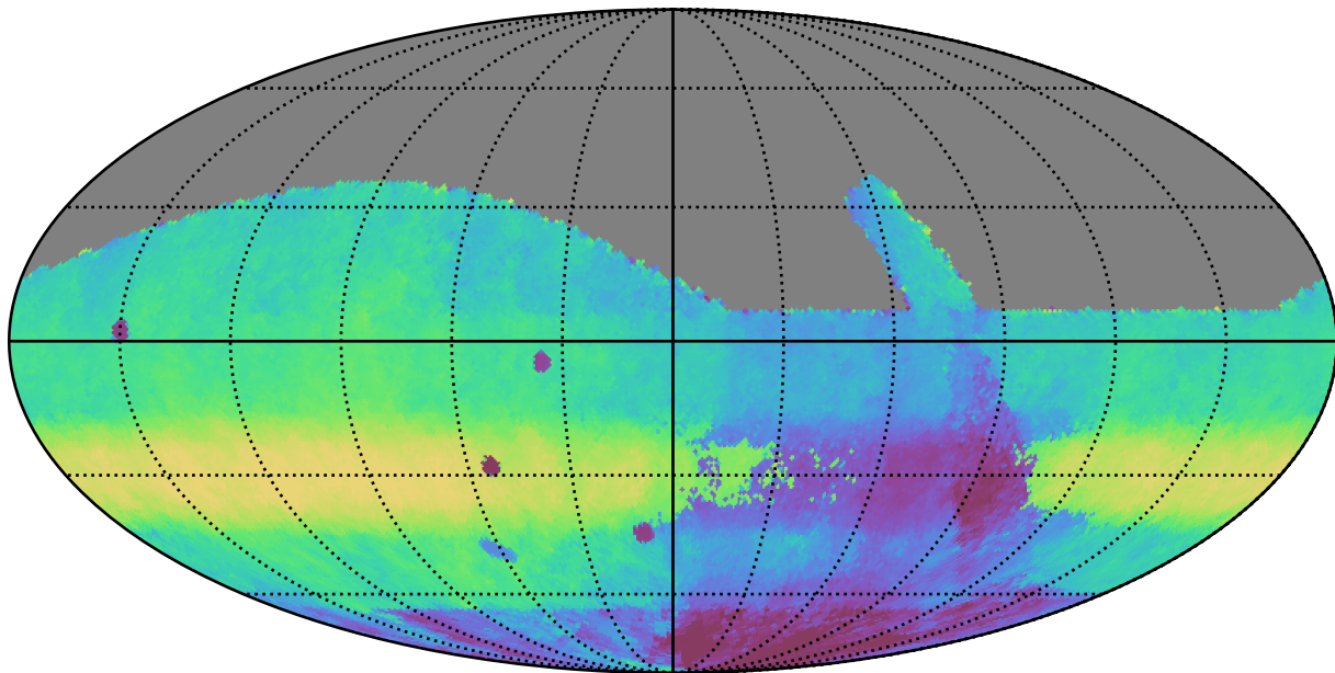
retro_baseline_v2.0_10yrs All sky i band: Median HA
