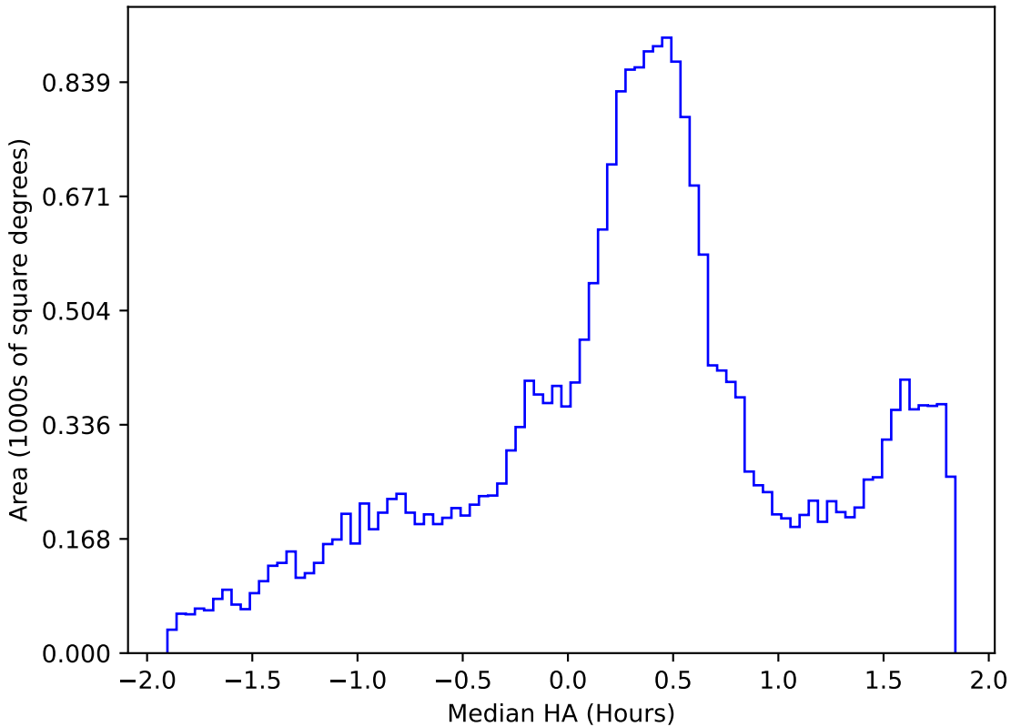
retro_baseline_v2.0_10yrs All sky i band: Median HA
