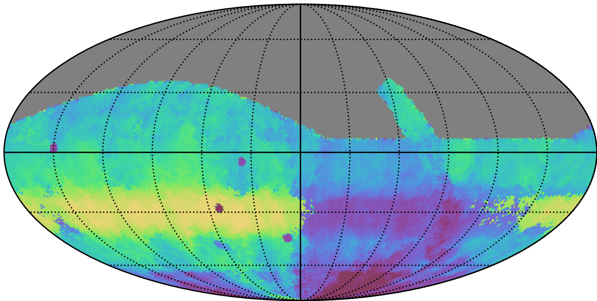
retro_baseline_v2.0_10yrs All sky g band: Median HA
