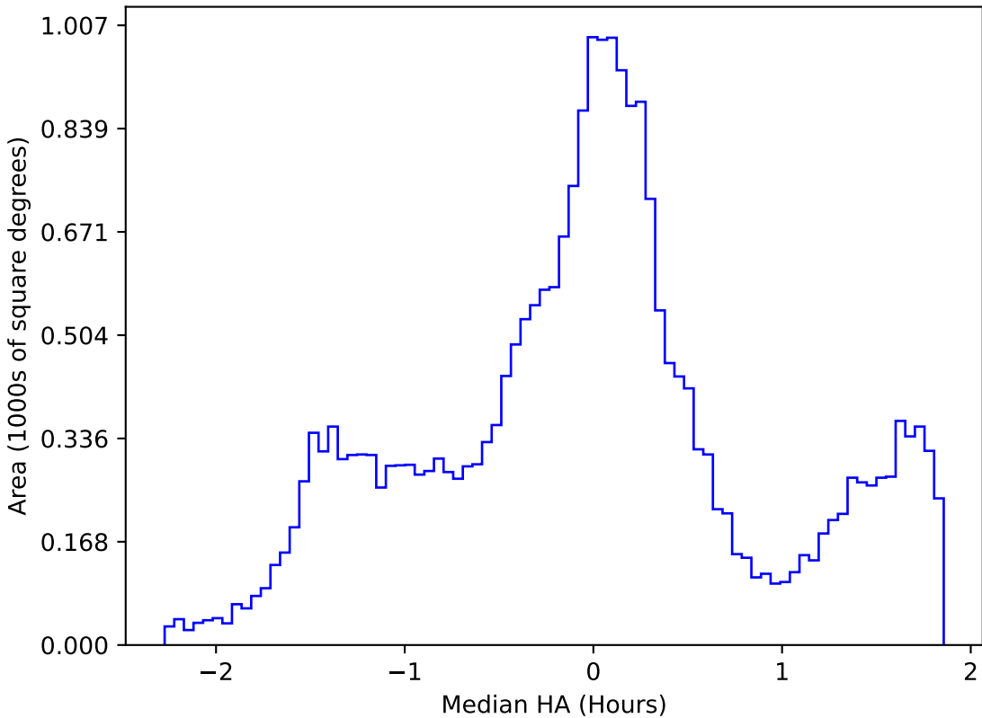
retro_baseline_v2.0_10yrs All sky g band: Median HA
