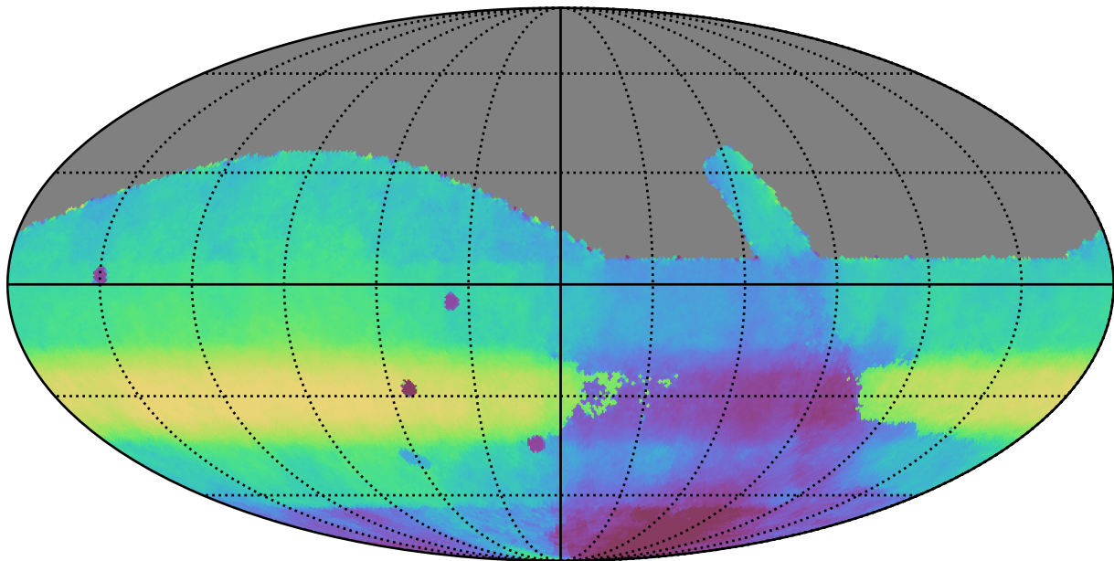
retro_baseline_v2.0_10yrs All sky all bands: Median HA
