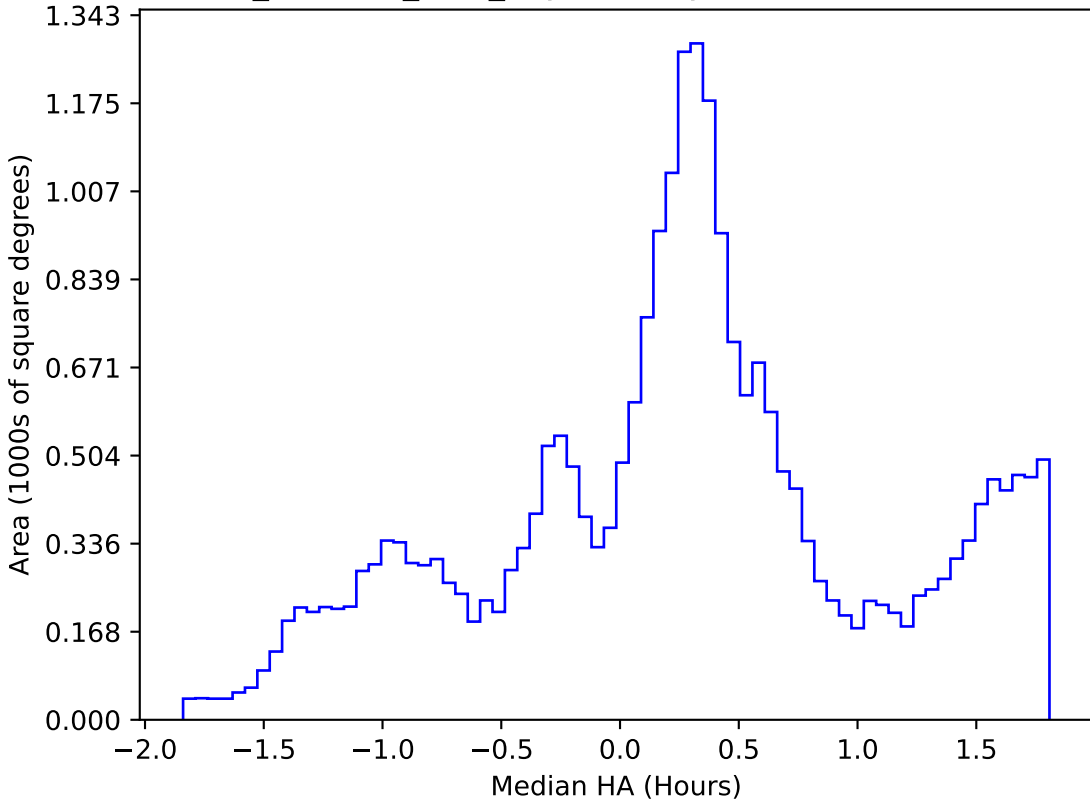
retro_baseline_v2.0_10yrs All sky all bands: Median HA
