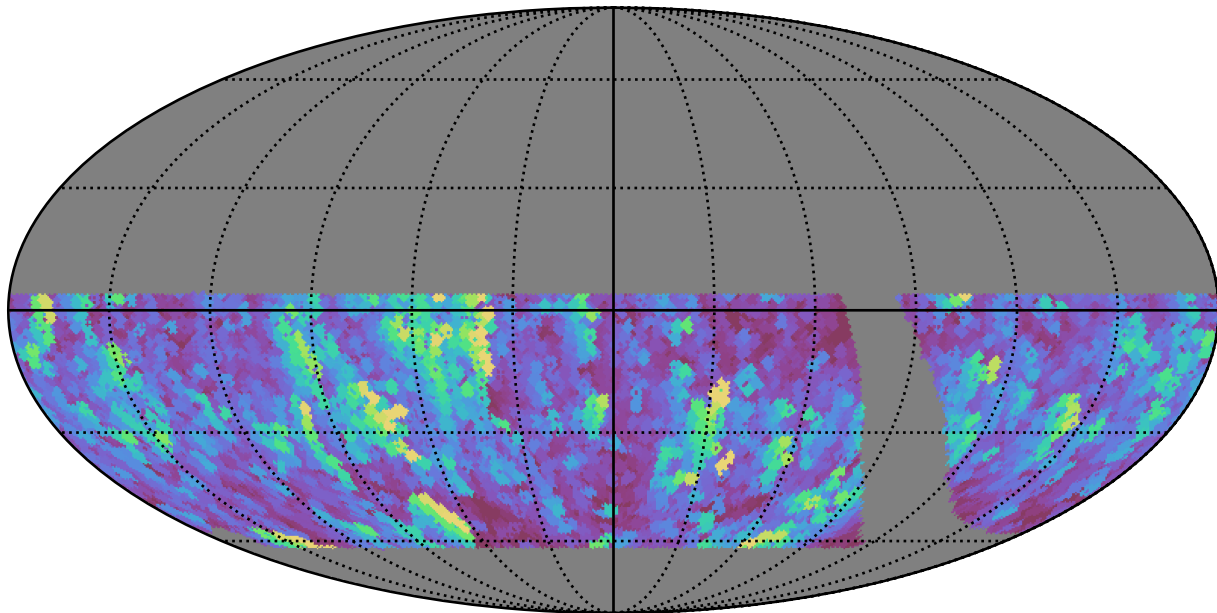
retro_baseline_v2.0_10yrs WFD y band: Max normairmass
