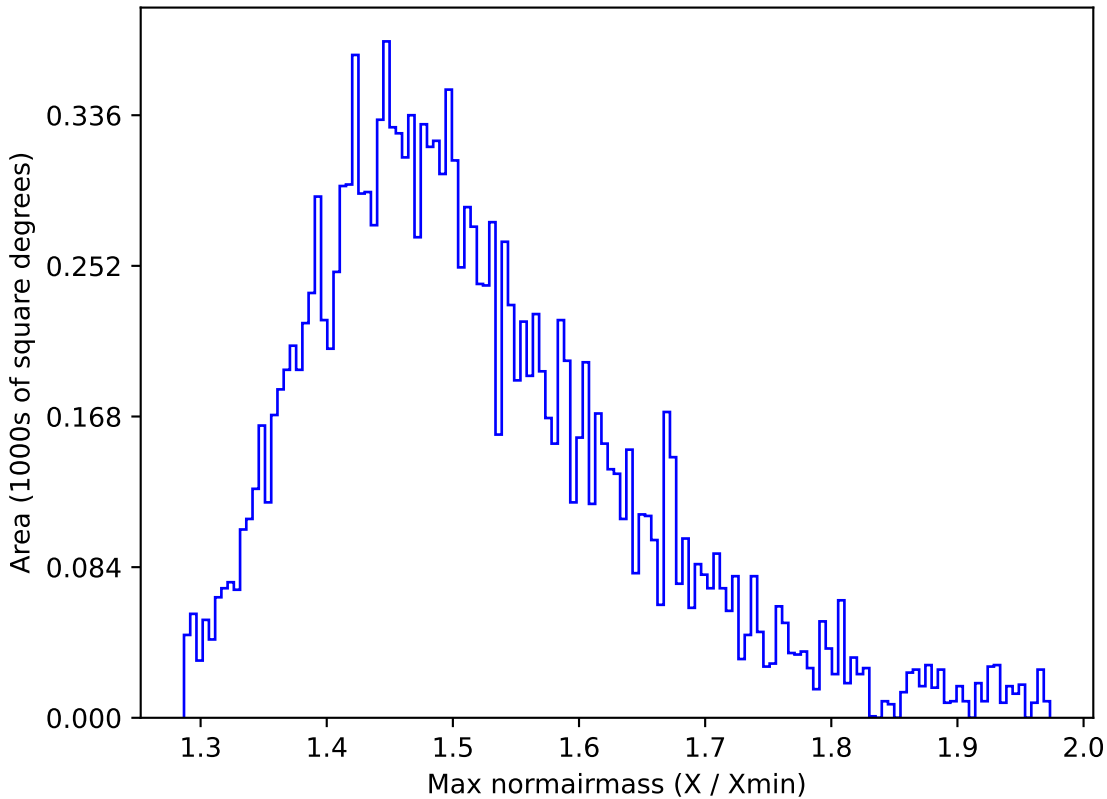
retro_baseline_v2.0_10yrs WFD y band: Max normairmass
