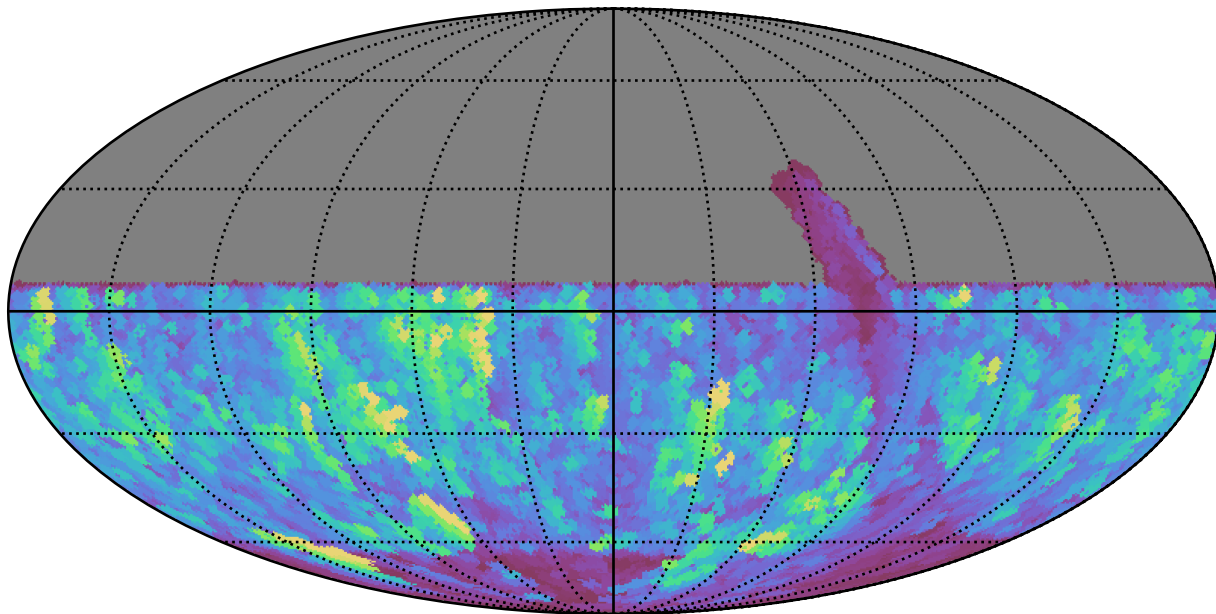
retro_baseline_v2.0_10yrs All sky y band: Max normairmass
