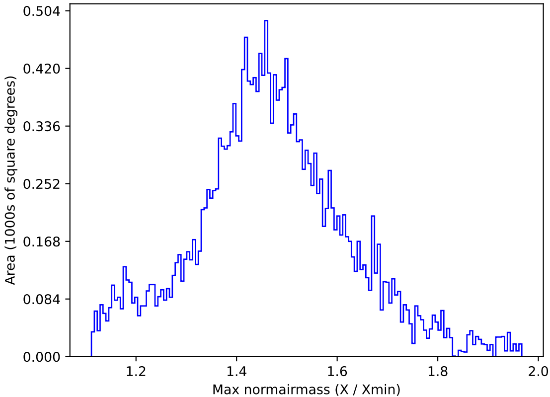
retro_baseline_v2.0_10yrs All sky y band: Max normairmass
