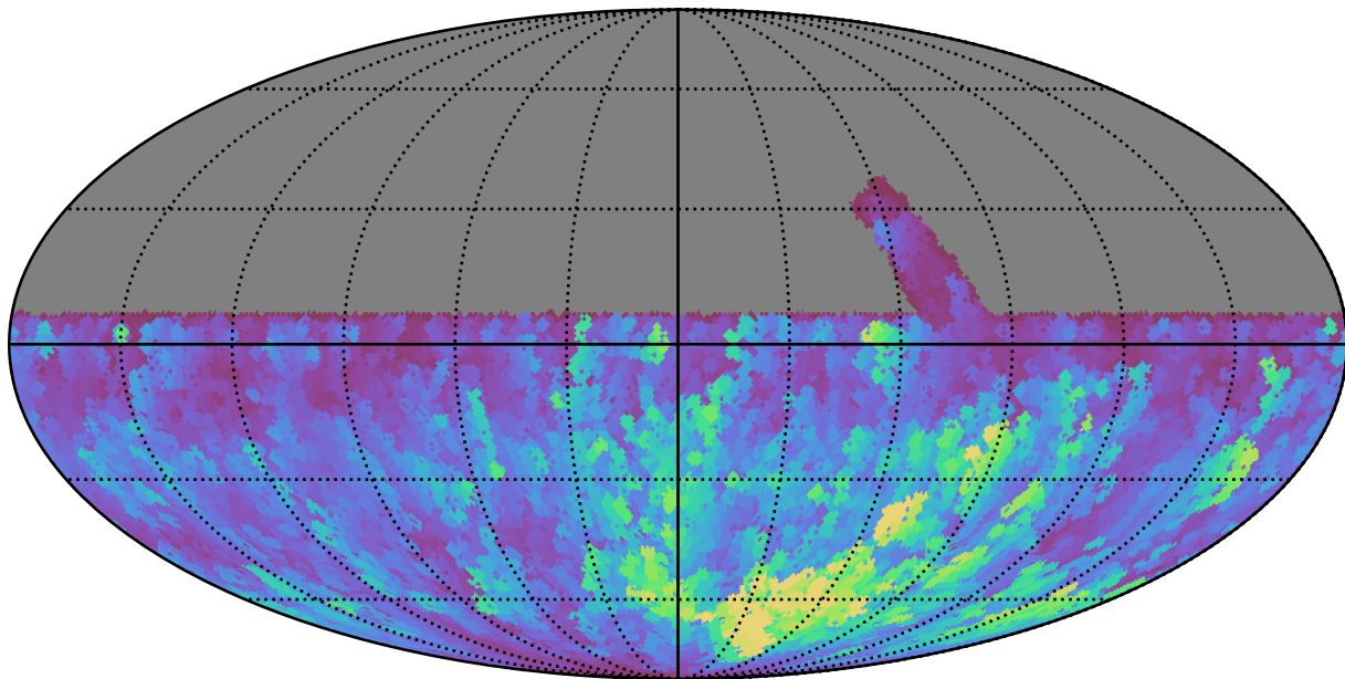
retro_baseline_v2.0_10yrs All sky u band: Max normairmass
