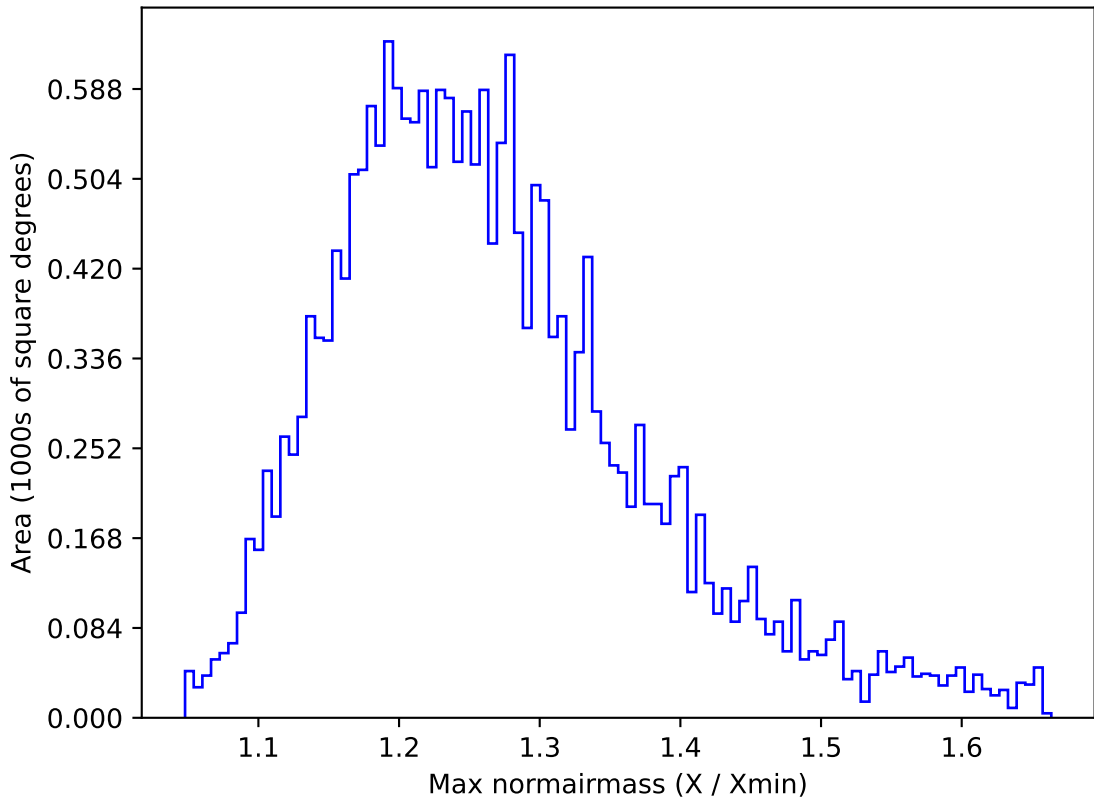
retro_baseline_v2.0_10yrs All sky u band: Max normairmass
