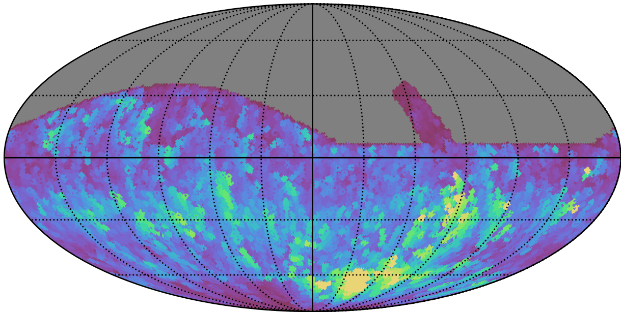
retro_baseline_v2.0_10yrs All sky r band: Max normairmass
